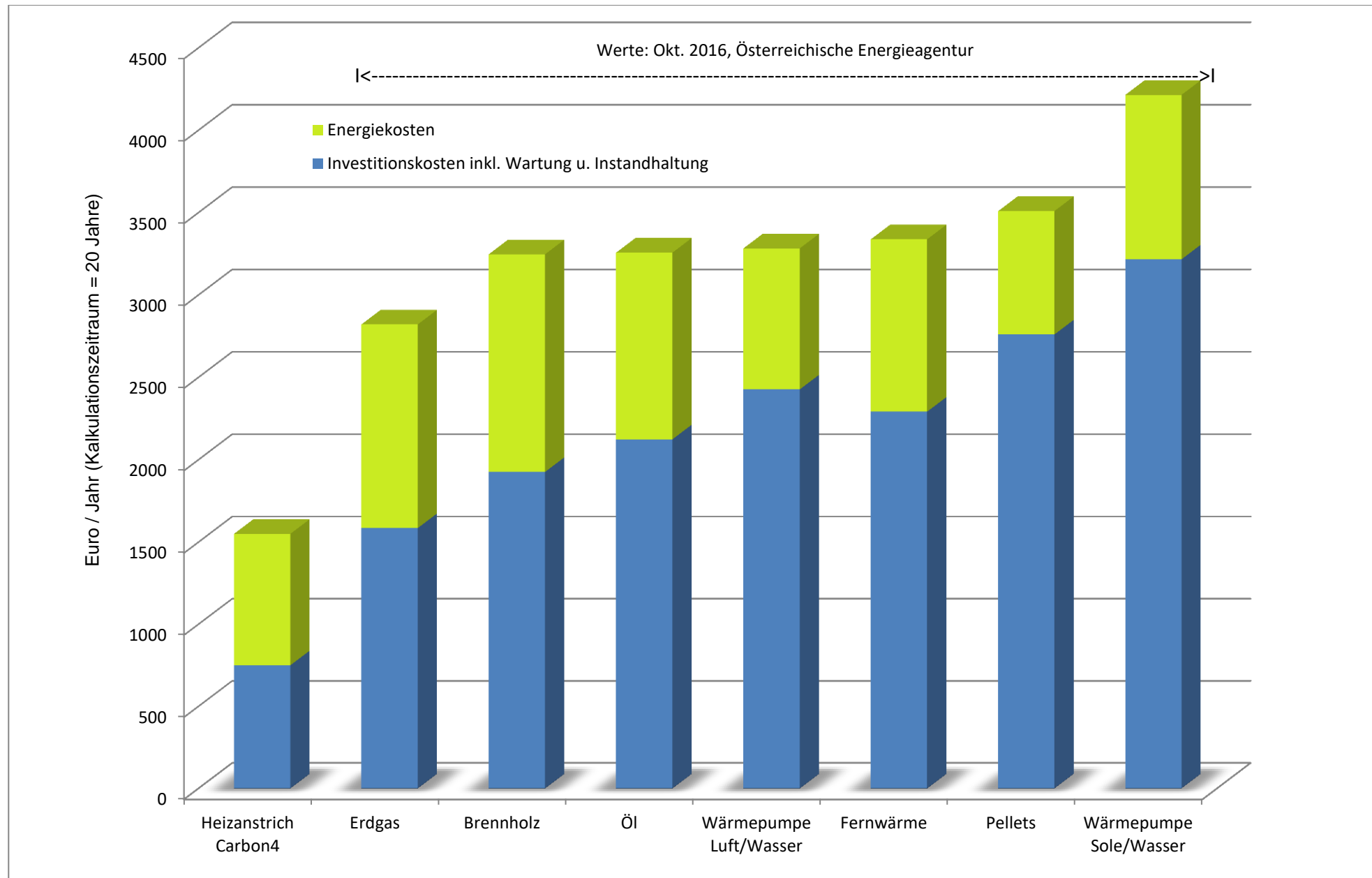
Investitions- und Energiekosten pro Jahr (Neubau, 118 m 2 Wohnfläche, Betrachtungszeitraum = 20 Jahre)
